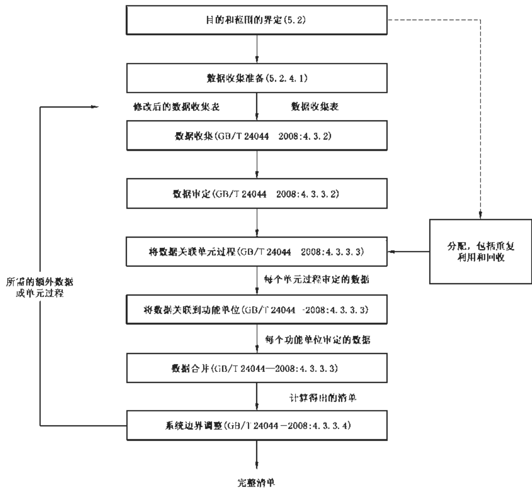
图 2 水足迹清单分析的简化流程
