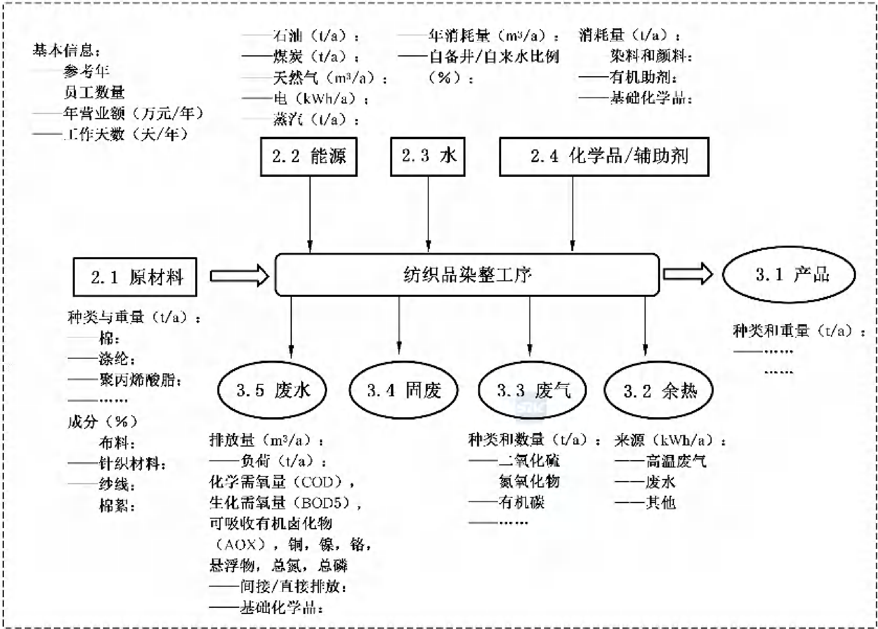
图 C.1 工序图:染整工序
